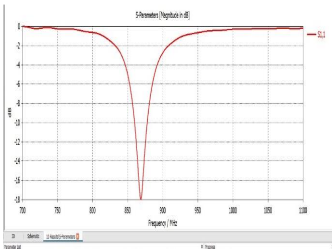
Fig. 4.2 S Parameter Result
