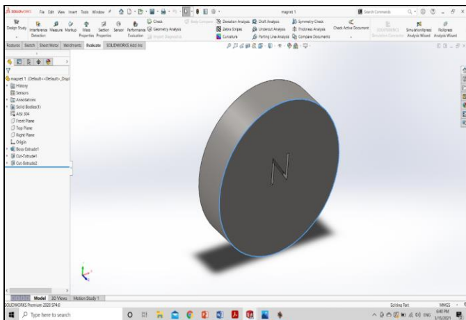
Fig 1 : Disc Magnet
