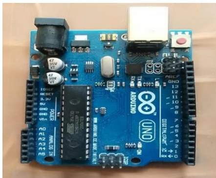
Fig. 4.1 Arduino Uno
