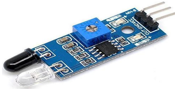
Fig.4 IR Sensor Module
