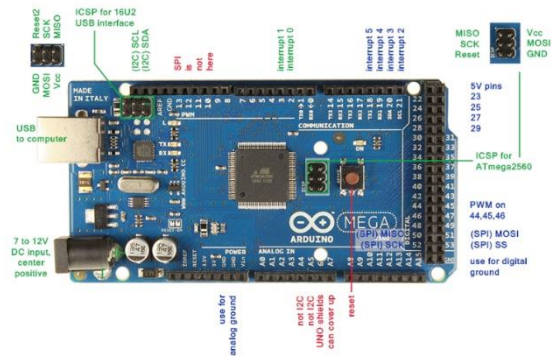
Fig 5.1 Arduino Mega
