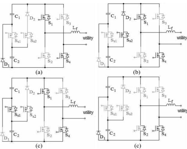
Fig. 3 Operation in the positive half cycle (a) mode 1 (b) mode 2 (c) mode 3 (d) mode 4
