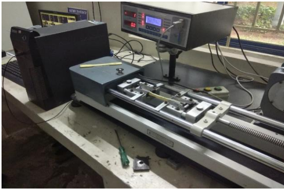
Fig 1.3 Tensile test
