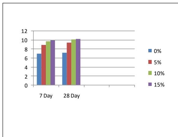
Fig. (d) Flexural Strength for M20 Grade Concrete
