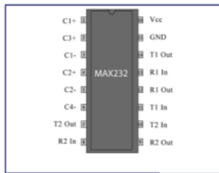
Fig 7. MAX232
