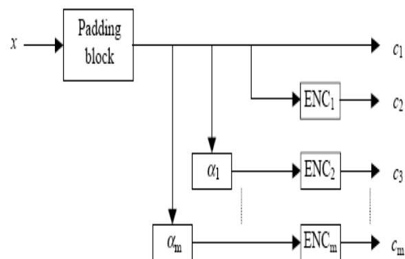
Fig. 1 turbo encoder
